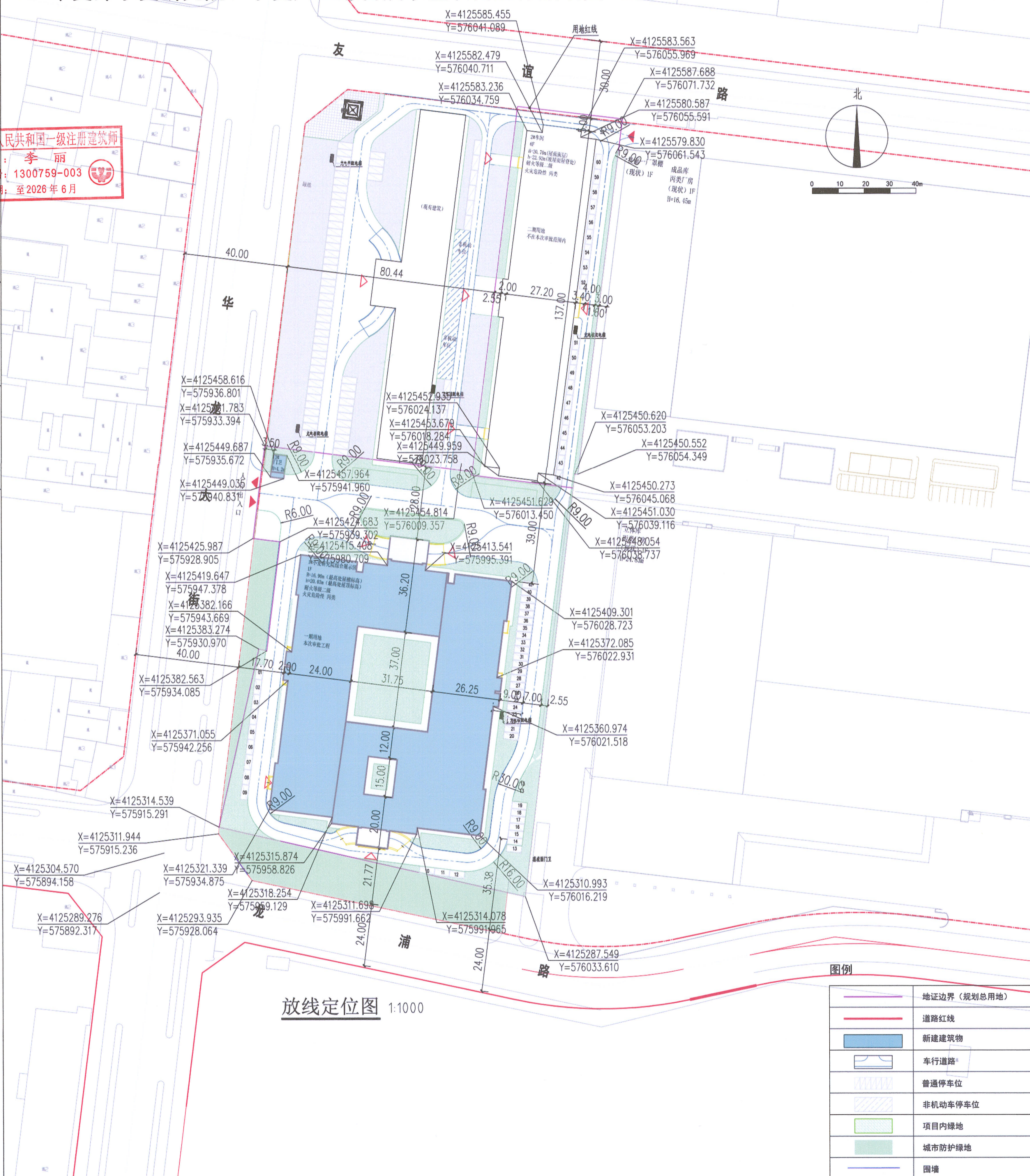
今麦郎小麦研究院、小麦产业综合展示区项目坐标放线图
